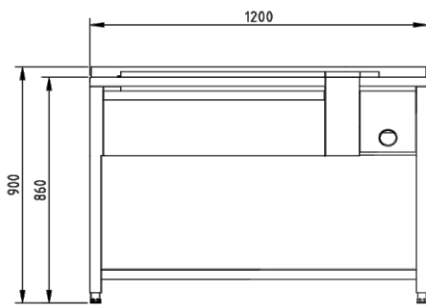
ALZADO
