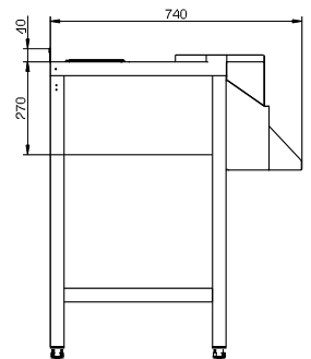
PERFIL
