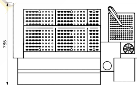
PLANTA CON SEGUNDO CARRIL RÁPIDO
