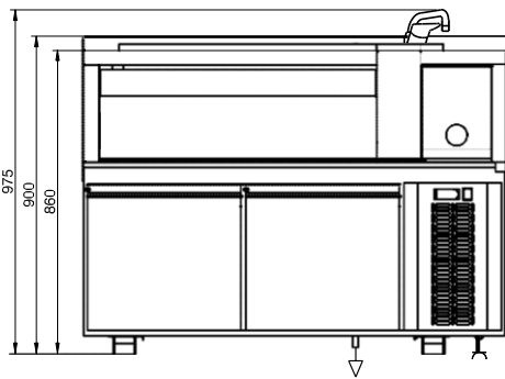
ALZADO
